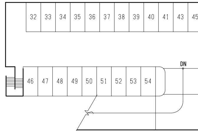
2階
